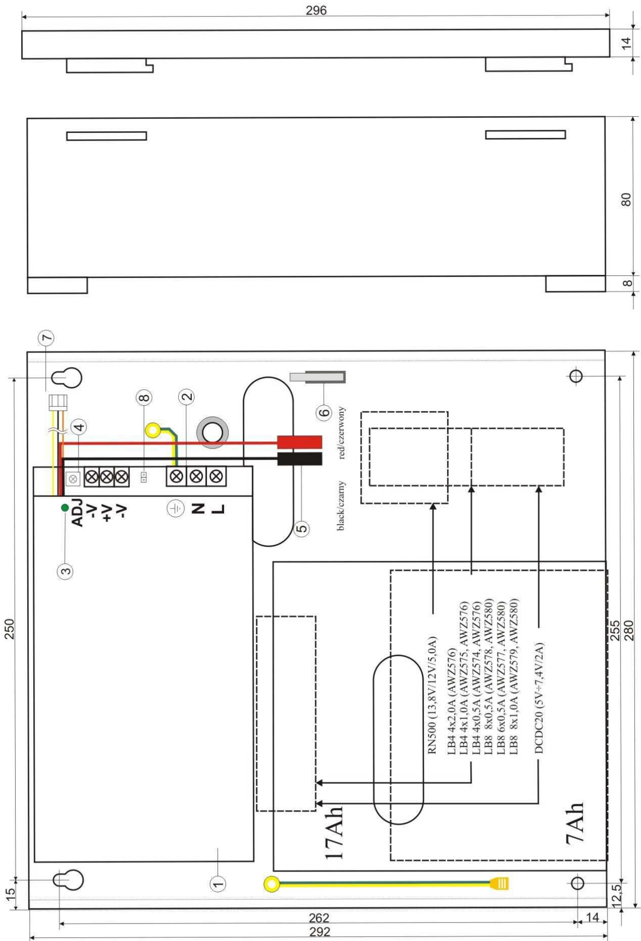
Rys.2. Widok zasilacza.
